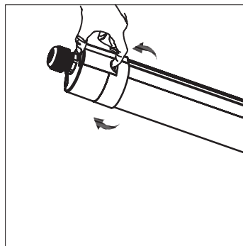
Gereedschaploze installatie
